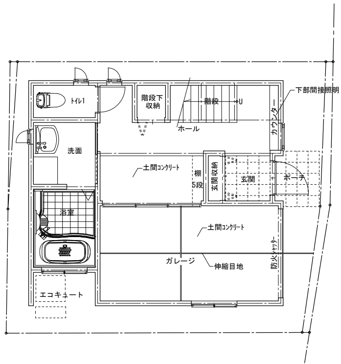
1階平面図兼配置図 S=1/100
