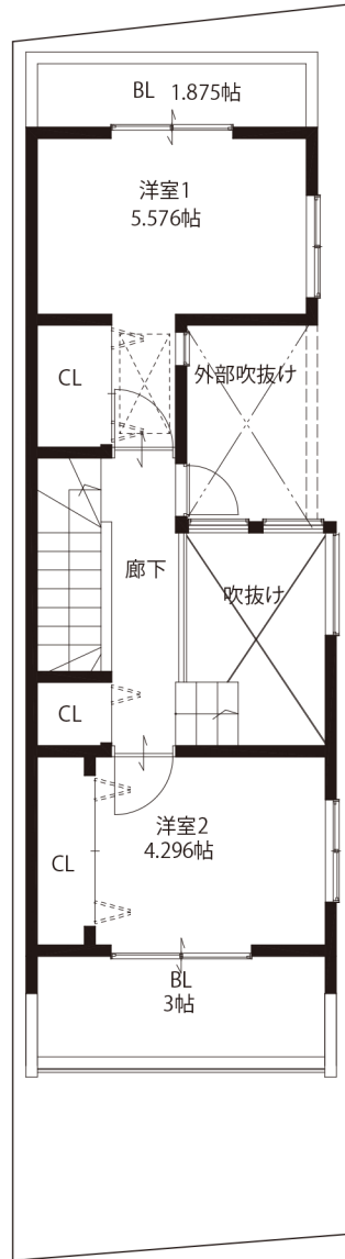
3階平面図
