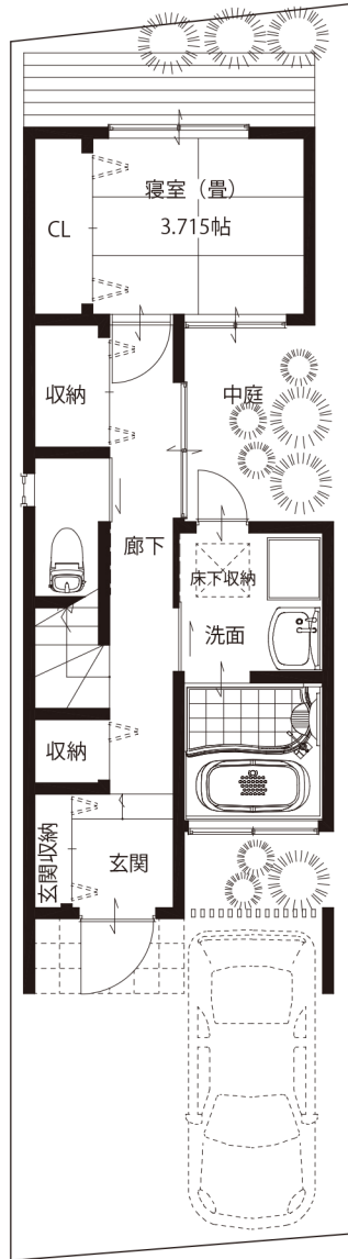
配置図兼1階平面図
