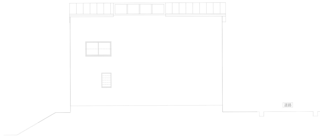
西侧立面图 1/100
