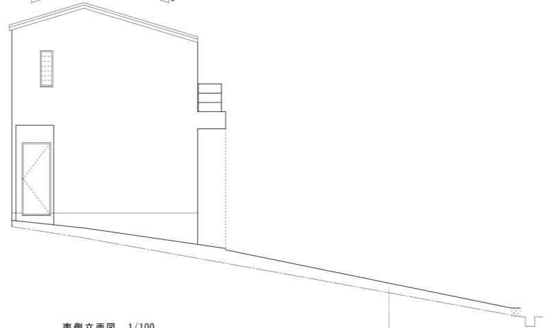
南侧立面图 1/100
