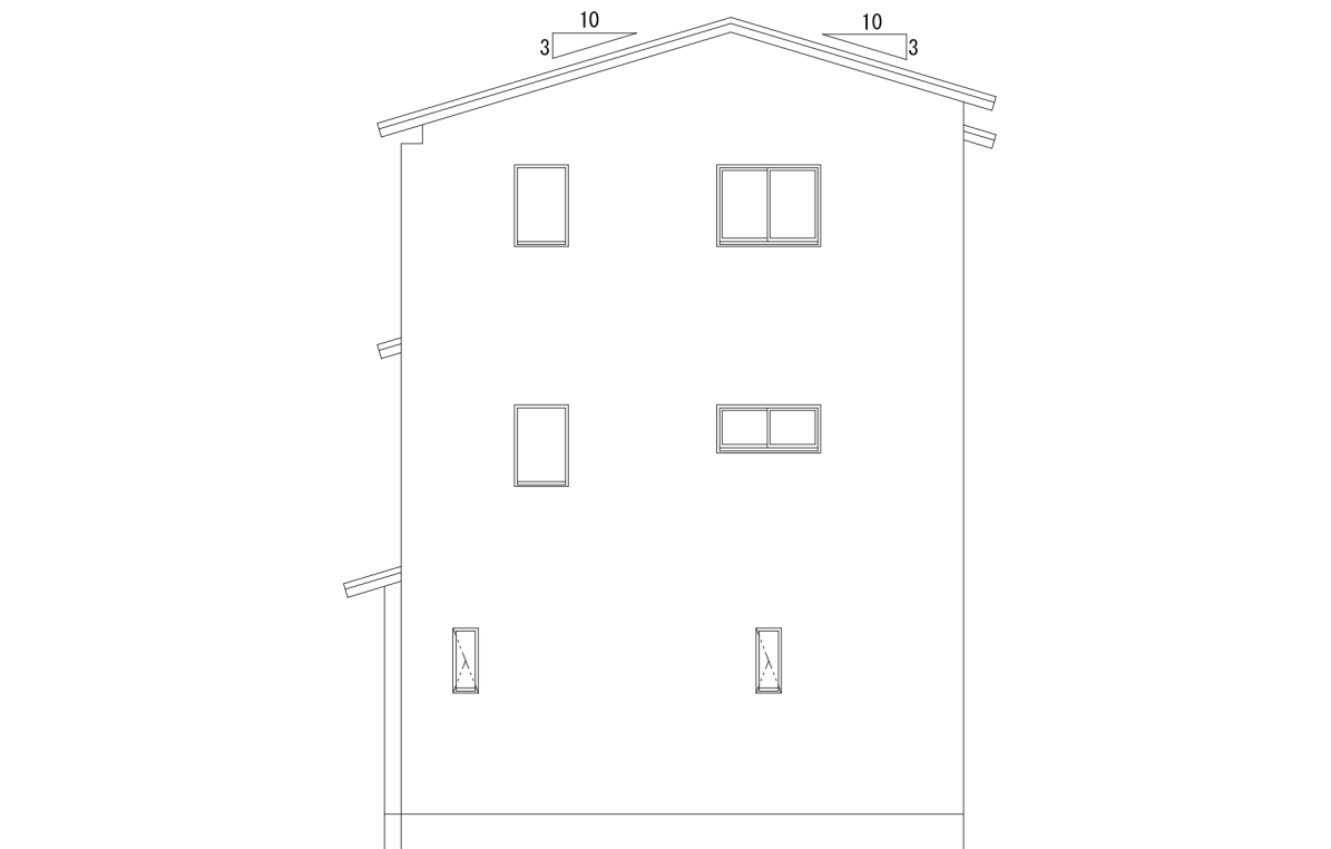
北立面图 S=1/100
