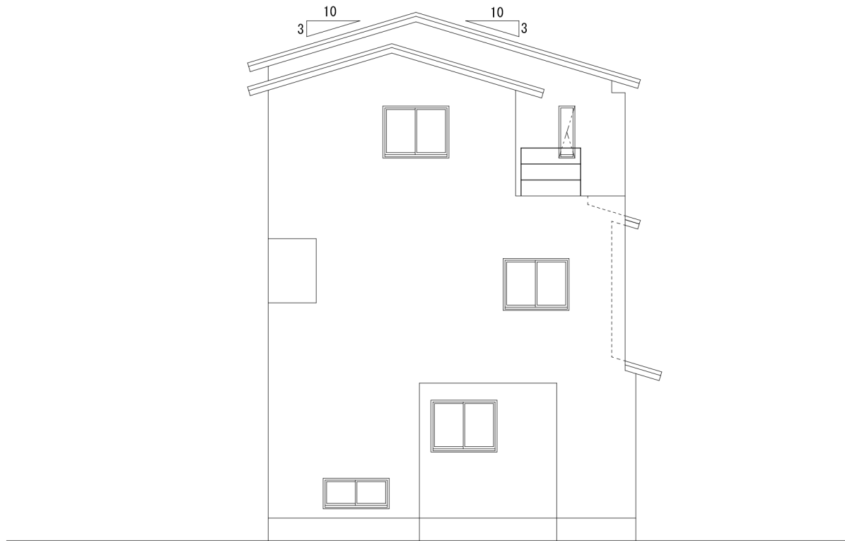
南立面图 S=1/100
