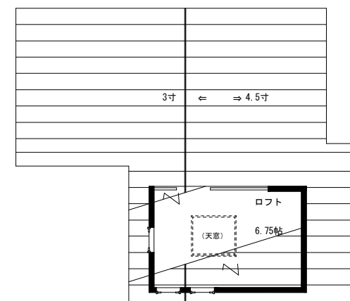
屋根伏図
